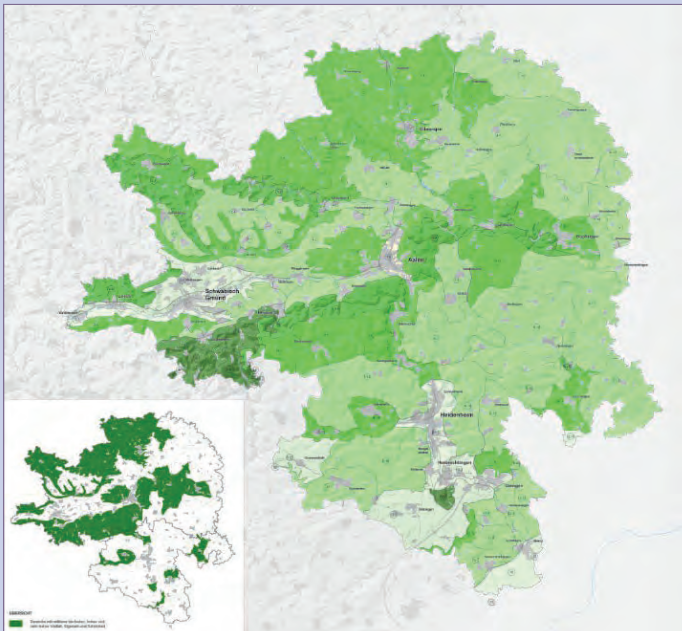
Flächendeckende Landschaftsbildbewertung
