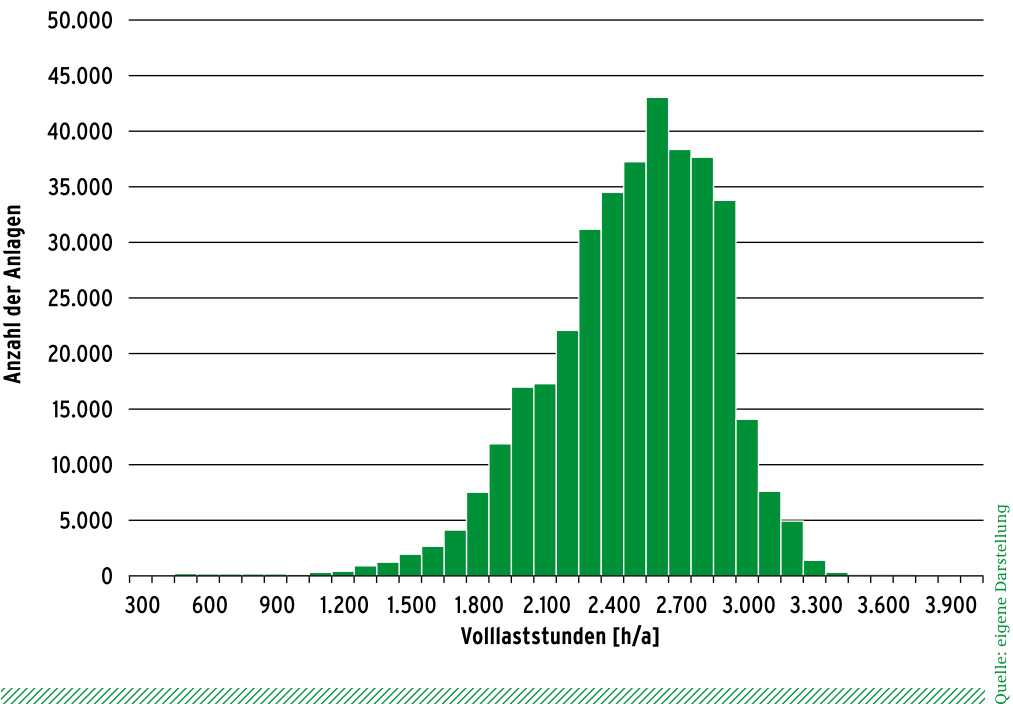
Abbildung 11: Häufigkeitsverteilung der Volllaststunden der Referenzanlagen im Bundesgebiet
