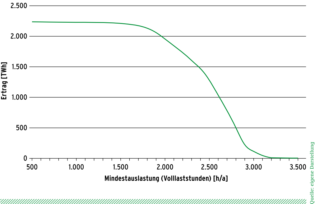
Abbildung 13: Potenzieller Ertrag aus Schwachwindanlagen in Abhängigkeit der Mindestauslastung (dargestellt ist ausschließlich der Ertrag aus Schwachwindanlagen)
