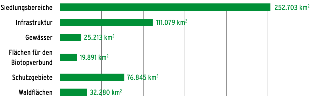
Abbildung 10: Ausschlusswirkungen der unterschiedlichen Flächenkategorien (Überschneidungen der Flächenkategorien wurden nicht berücksichtigt)
