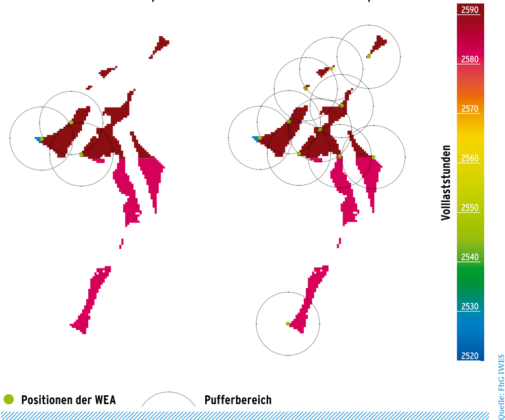
Abbildung 8: Positionen der ersten drei WEA innerhalb eines Windparks
