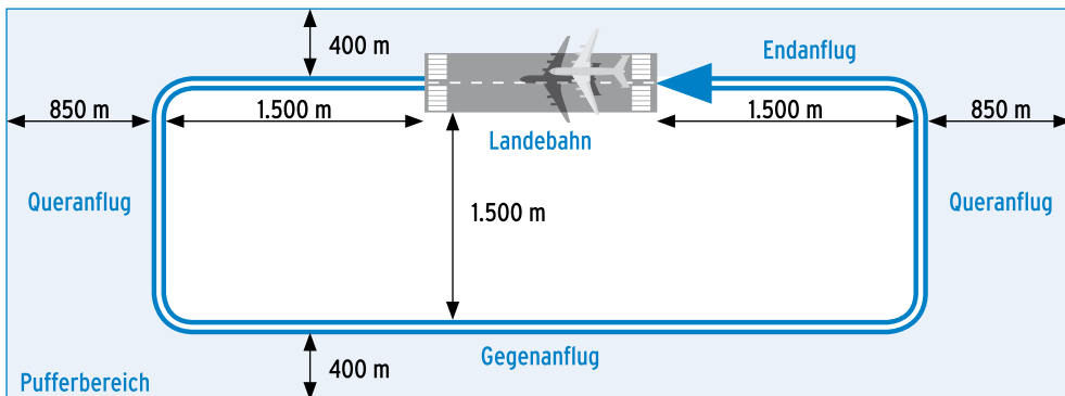
Abbildung 6: Ausschlussflächen bei der Genehmigung von WEA im Umfeld von Flugplätzen
