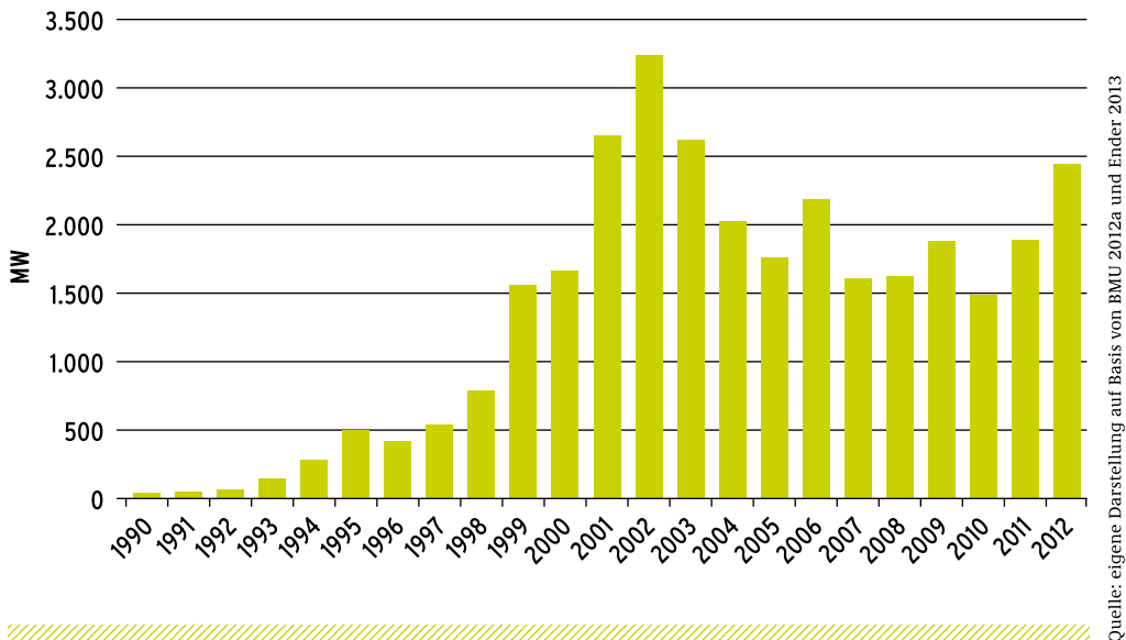
Abbildung 1: Entwicklung der jährlich neu installierten Windenergieleistung (Rückbau aufgrund von Repowering nicht berücksichtigt)
